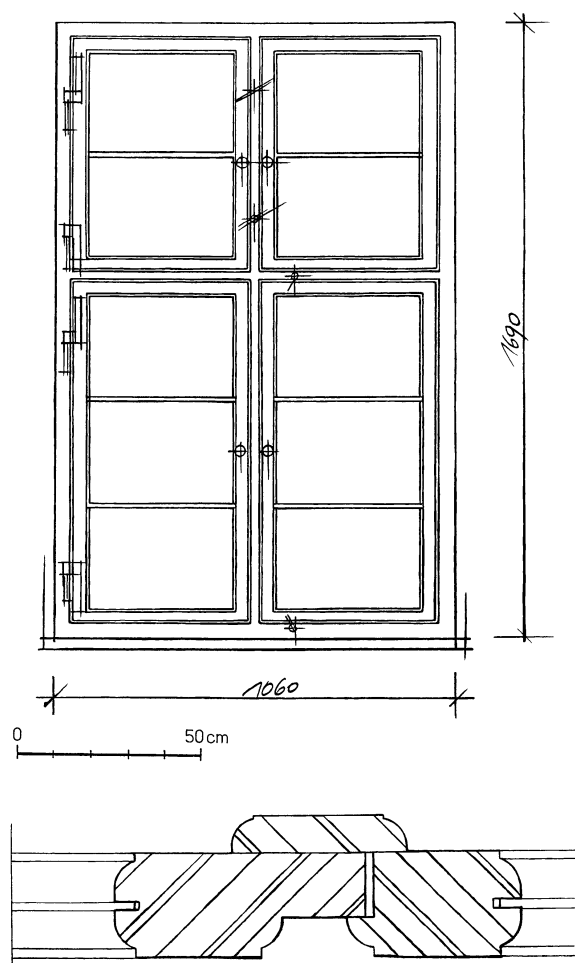
Obr. 15: Sádek čp. 33 – dům, okno v jihovýchodní stěně světnice v přízemí (zaměření a kresba P. Dostál).
