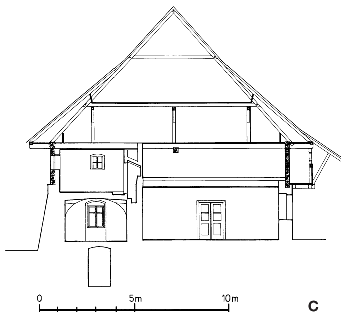
Obr. 6: Sádek čp. 33, časové zařazení stavebních konstrukcí: A – dům, patro (21 – síň, 22 – horní světnička, 23–25 – komory) (zaměření P. Šafář, kresba R. Ahneová); B – sklep (zaměření P. Šafář, kresba R. Ahneová); C – dům, příčný řez (zaměření P. Šafář, kresba P. Dostál).
