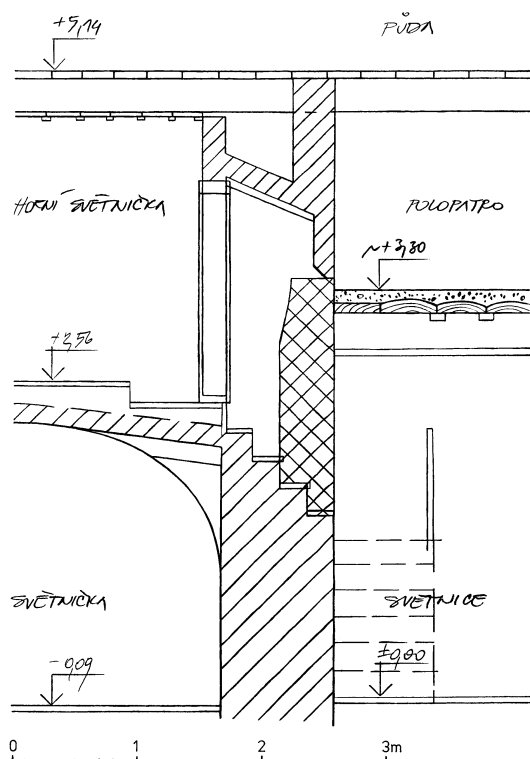
Obr. 7: Sádek čp. 33 – dům, detail příčného řezu v místě vstupu do horní světničky (kresba P. Dostál).
