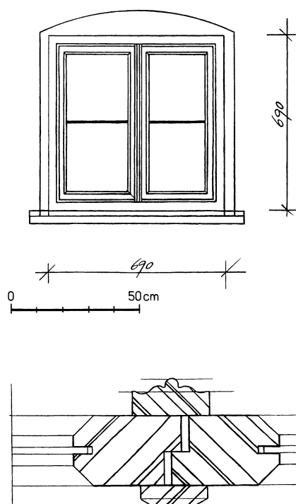
Obr. 16: Sádek čp. 33 – dům, okno v severovýchodní stěně světničky v patře (zaměření a kresba P. Dostál).
