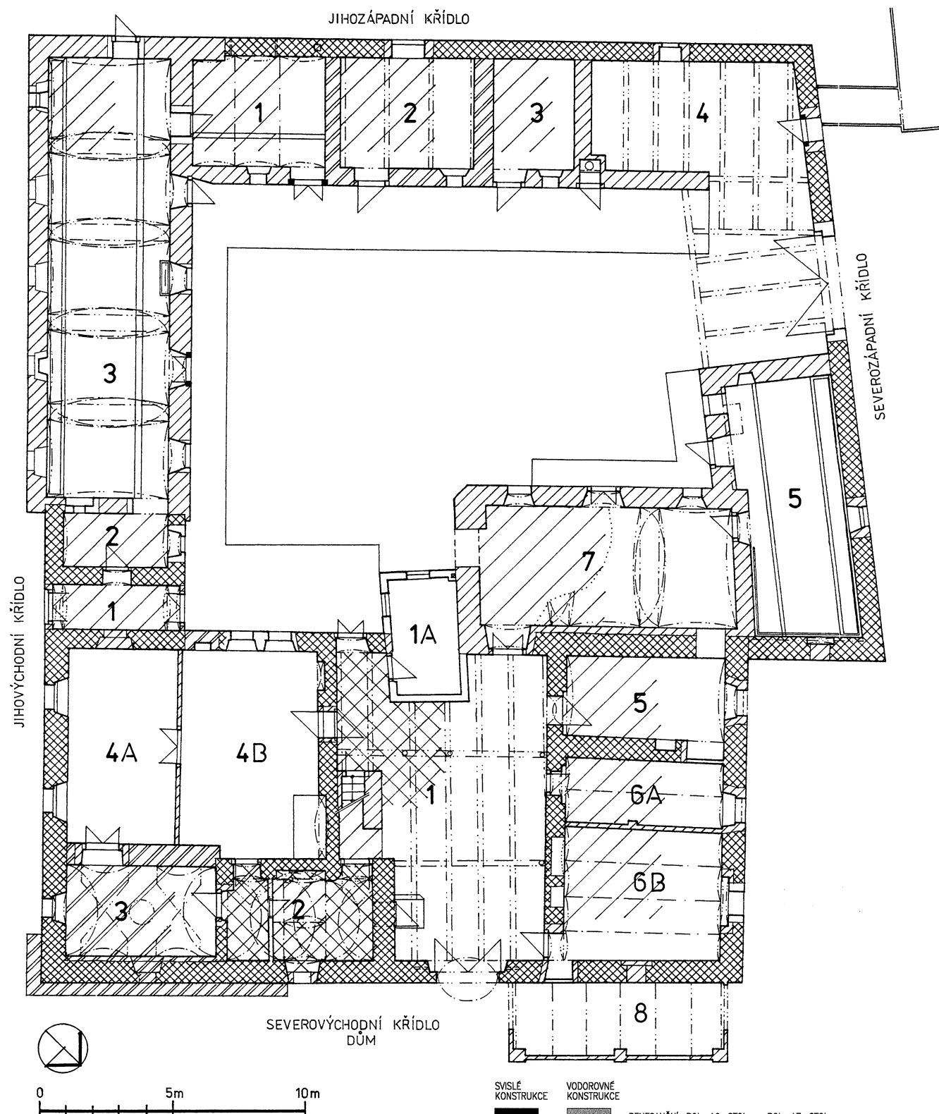
Obr. 5: Sádek čp. 33, časové zařazení stavebních konstrukcí – přízemí (dům 1 – síň, 2 – kuchyně, 3 – světnička, 4 – světnice, 5, 6 – komory, 7 – stáj pro koně, 8 – přístavek; jihovýchodní křídlo 1 – chodba, 2 – přípravná, 3 – chlév; jihozápadní a severozápadní křídlo 1–3 – stáj, 4 – kolna, 5 – stáj) (zaměření P. Šafář, kresba R. Ahneová).
