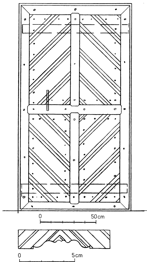
Obr. 17: Sádka čp. 33 – dům, vnější dveře světnice v přízemí (zaměření R. Ahneová, kresba P. Dostál).
