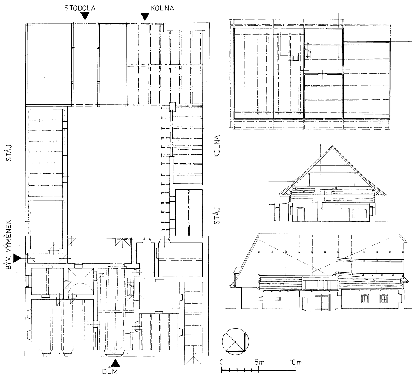
Obr. 37: Sádka čp. 26 – dispoziční schéma přízemí usedlosti a patra domu, příčný a podélný řez domem (zaměření a kresba R. Ahneová, P. Dostál).
