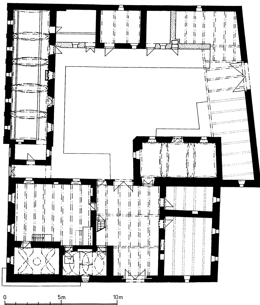
Obr. 36: Sádka čp. 33 – přízemí, rekonstrukce stavu po roce 1856 (kresba P. Šafář).
