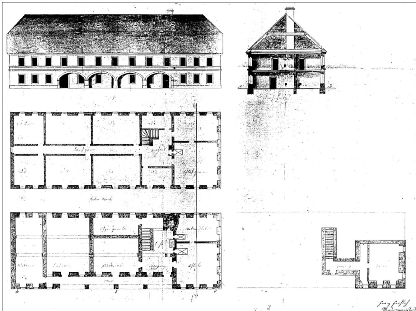
Obr. 5: Louboř, projekt nové výstavby domu největší usedlosti čp.1: Plan... (?) den N. N. Bauergutts besitzer in Lauben No zur widererbauung des abgebrannten Wunhauses, s. d. (přelom dubna a května 1843), zednický mistr Franz Fröhlich, půdorysy sklepa, přízemí a 1. patra, pohled, řez (SOBA Děčín, Vs Česká Lípa, kt. 252, plán 7). Značení kleneb v přízemí je schématické, jenom pomocí dělicích pasů, dlouhá boční fasáda je členěná jenom odlišným rytmem okenních os, zdůrazněným ve střední části čtveřicí arkád, chránících hospodářskou komunikaci. Jasně je vyznačení otopného zařízení s velkou chlebovou pecí a ještě nepřímo vytápěnými kamny.
