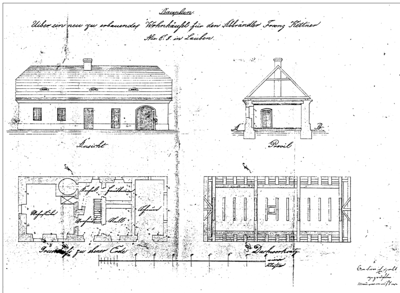
Obr. 17: Loubí, projekt na stavbu chalupy čp. 8: Bauplan ein neu zu erbauendes Wohnhaußel für den Abbrändler Franz Kettner Nro C. 8 in Lauben, s. d. (1843), zednický mistr Anton Eiselt, graf. měř. vídeňské sáhy, půdorys přízemí, pohled, řez, vazba (SOBA Děčín, Vs Česká Lípa, kt. 252, plán 5). Stavba byla provedena dosti odlišně - jako patrová, ve zděné části kratší, jenom trojdílná (napojený díl stodůlky je dřevěný). Odlišné je i provedení zadní kuchyňské části síně, která je celá oddělena klenutým pasem.
