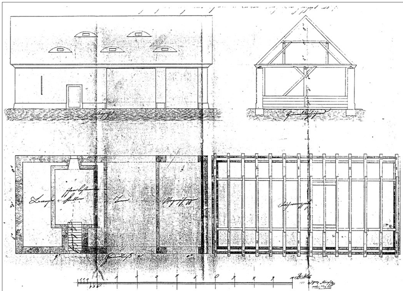
Obr. 16: Loubo, projekt na stavbu stodoly v usedlosti čp. 7: Bauplan zur herstellung einer Scheuer in Lauben, Neuschlosser Herrschaft No 7, s. d., zednický mistr Ignác Kriesch, grafické měřítko vídeňské sáhy - půdorys, pohled, řez, vazba (SOBA Děčín, Vs Česká Lípa, kt. 252, plán 11). Objekt se dochoval ve stavu, dokládajícím důsledné provedení stavby podle projektu (např. včetně počtu a tvaru vikýřů).
